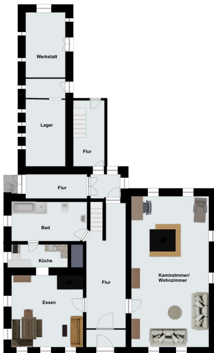
Erdgeschoss
